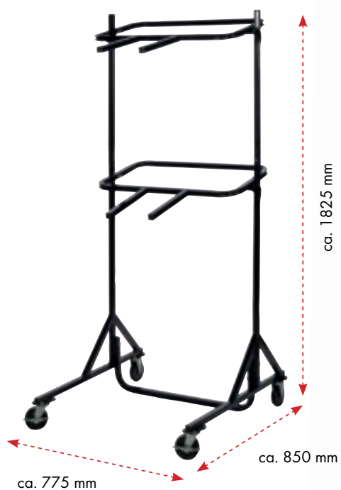
POS SCHUBKARREN- PRÄSENTATIONSSTÄNDER
